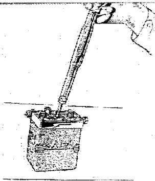
Fig. 7 - Misura della carica della batteria con densimetro Control of the battery charge by means of densimeter
