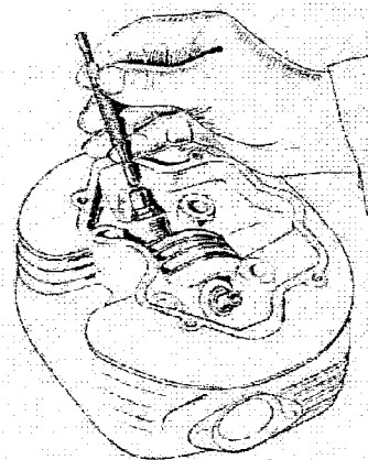
Fig. 12 - Controllo dei fori delle guide delle valvole Checking the holes of the valve guides.
