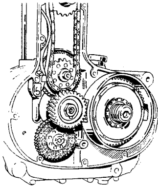
Fig. 25 - Attrezzo di blocco per smontaggio e montaggio del dado pignone motore Securing tool for disassembling and assembling the engine pinion nut
