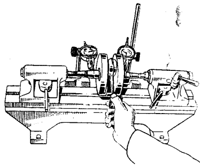
Fig. 30 - Controllo dell'allineamento del volano motore FLY WHEEL RIM ALIGNMENT
