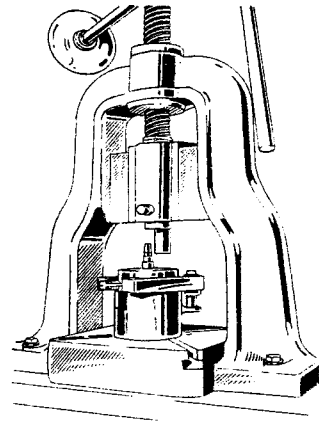
Fig. 28 - Disaccoppiamento del volano motore Decoupling the engine flywheel.
